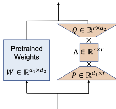
(b) AdaLoRA
